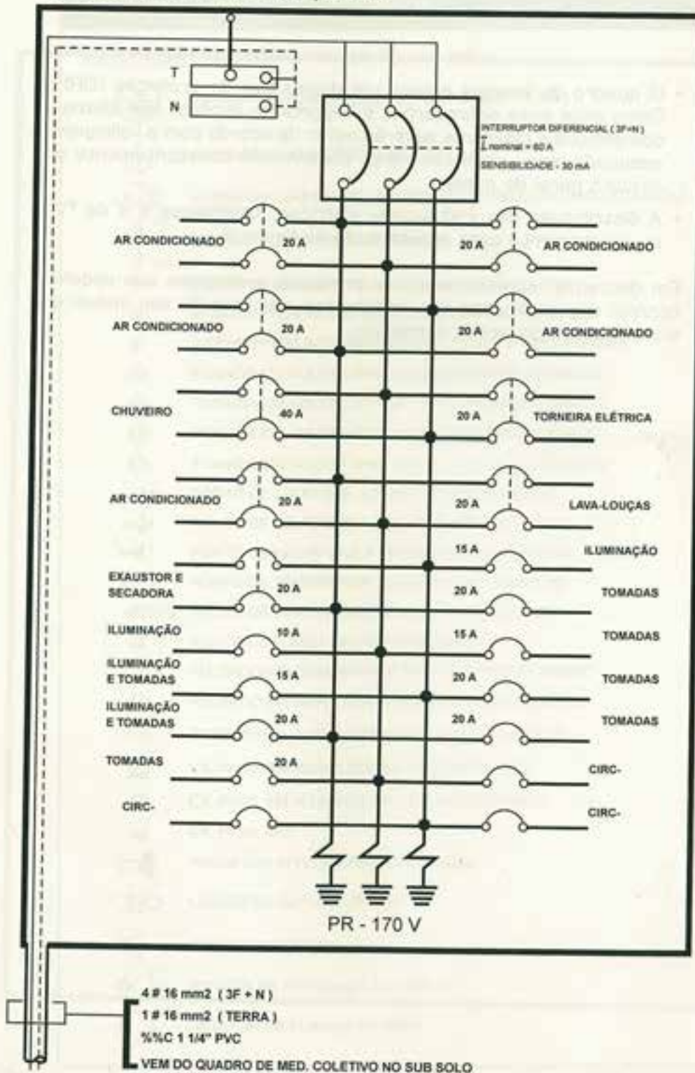
QL. APTO. TIPO - 127/220V
